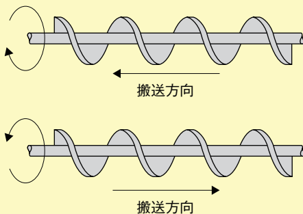
右巻スパイラー (R)
